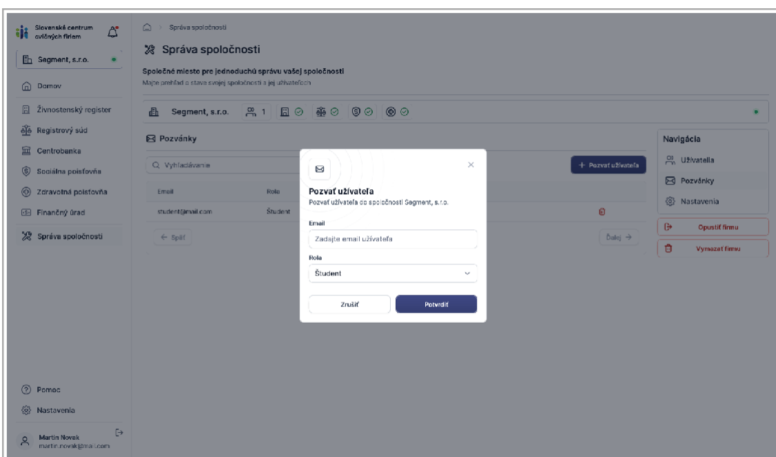
Obrázok 63: Pozvanie užívateľa
